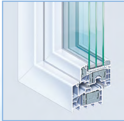
EGE 88plus mit Thermoeinschüben – zertifiziert vom Passivhausinstitut Dr. W. Feist
