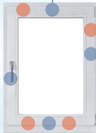
entspr. WK 1 mit abschließbarem Handhebel
